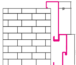
Opaska z ościeżnicą wewnętrzną IRON
