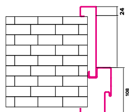
Opaska z ościeżnicą regulowaną IRON
